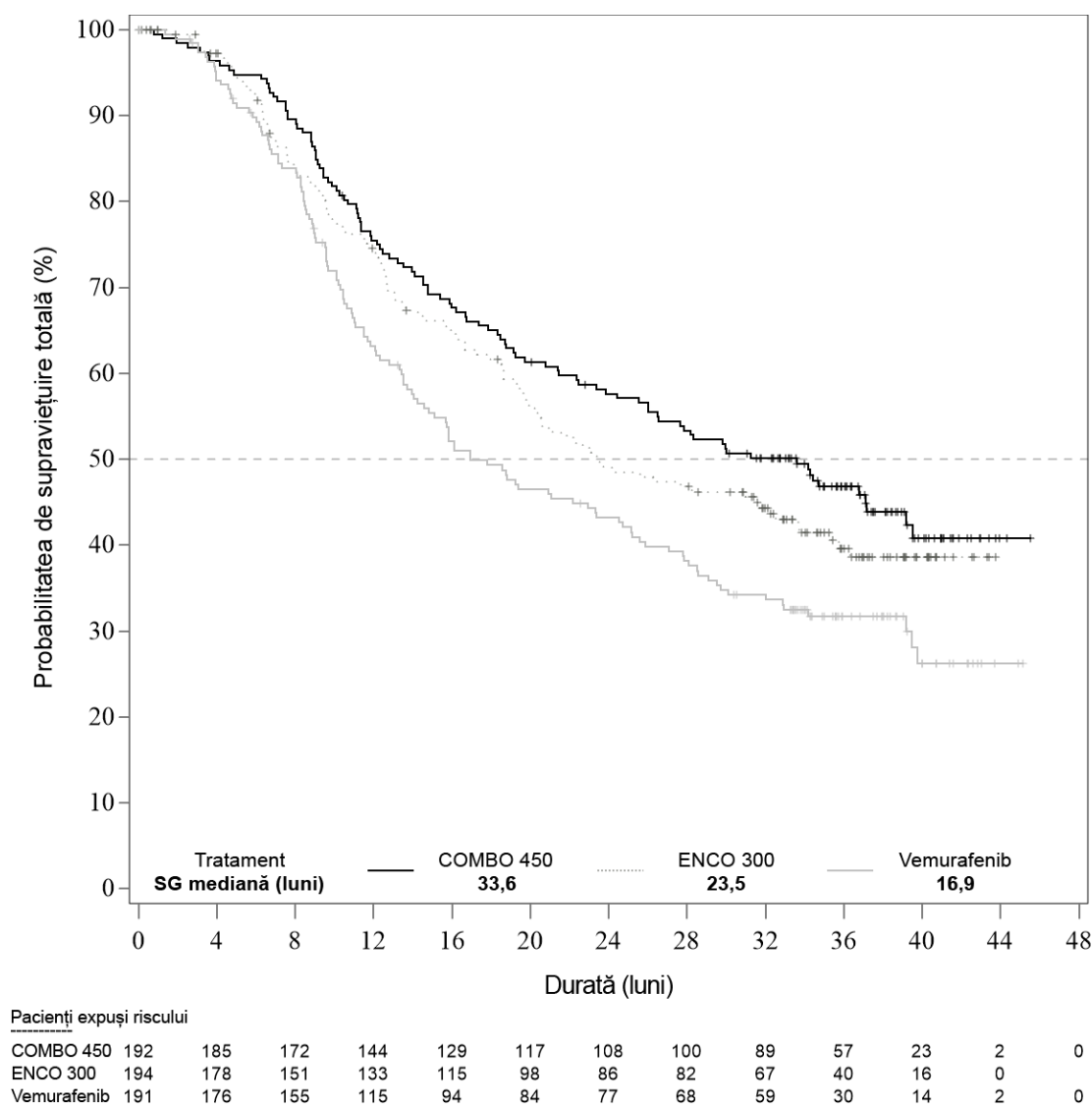
Figura 2 Studiul CMEK162B2301, Partea 1: Reprezentare Kaplan-Meier a supraviețuirii generale, rezultate intermediare (data-limită a colectării datelor: 7 noiembrie 2017)
